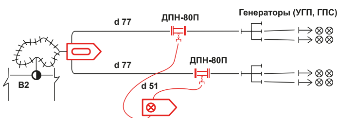
Схема подключения ДПН-80П
