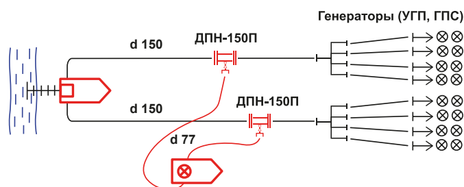
Схема подключения ДПН-150П
